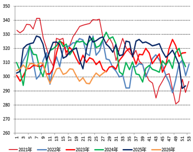
图10 热卷周产量
